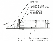
7 DOOR JAMB AT GWB 1 1/2\"/>
