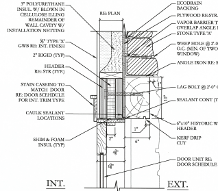
2 DOOR HEAD AT STONE 1 1/2\"/>
