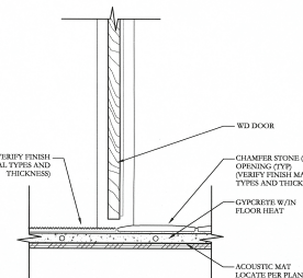
11 DOOR SILL AT GWB 1 1/2\"/>
