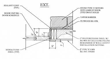
6 DOOR JAMB AT STONE 1 1/2\"/>
