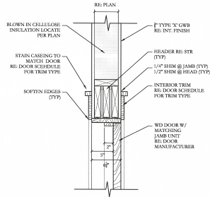
3 DOOR HEAD AT GWB 1 1/2\"/>
