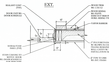
5 DOOR JAMB AT SIDING 1 1/2\"/>
