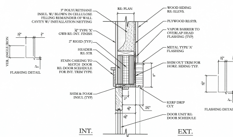
1 DOOR HEAD AT SIDING 1 1/2\"/>
