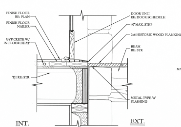
10 DOOR SILL AT STONE 1 1/2\"/>
