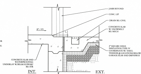
12 GARAGE DOOR SILL AT STONE 1 1/2\"/>
